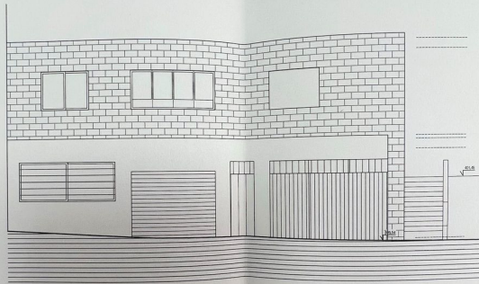
ALZADO OESTE
