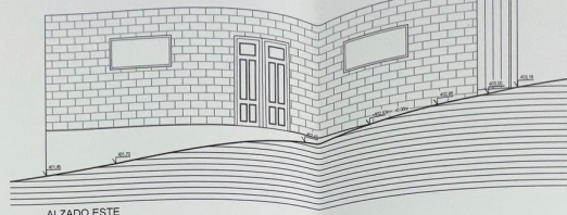
ALZADO ESTE
