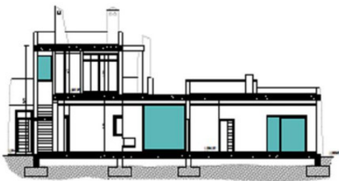
SECCIÓN A-A'
