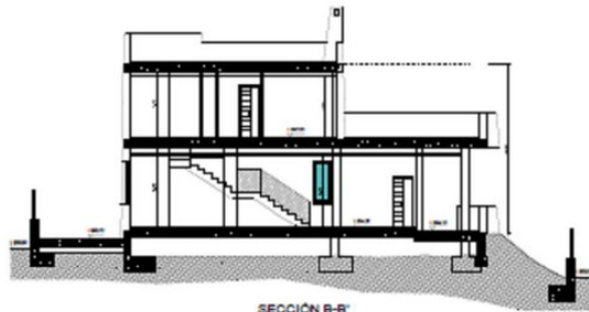
SECCIÓN B-B'
