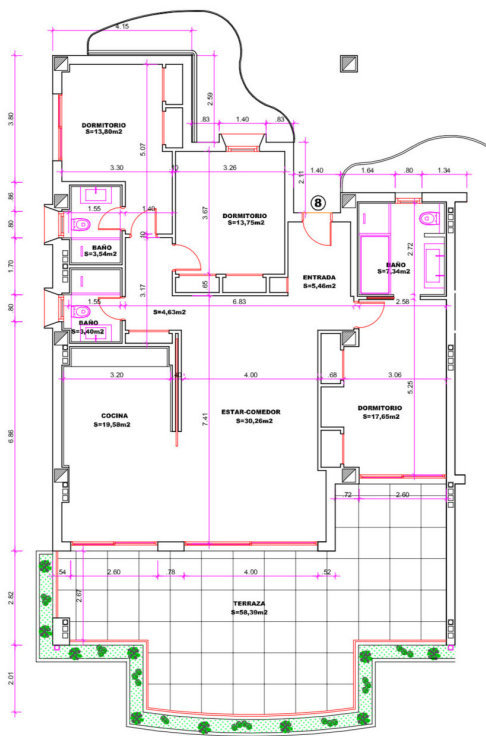
Apartamento 8 Escala 1:100
