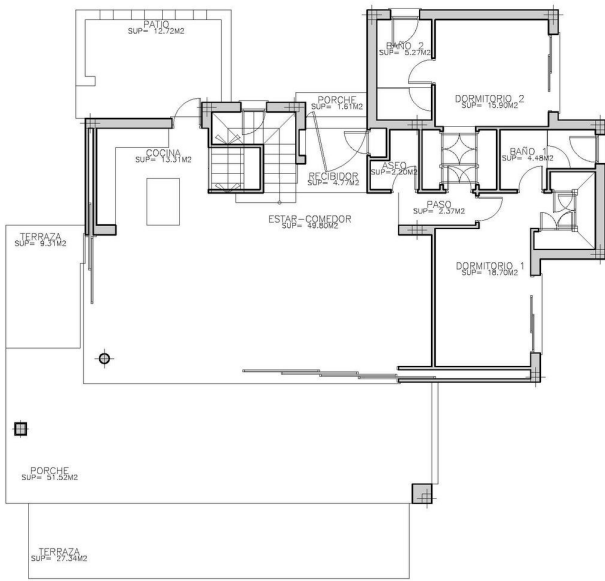
PLANTA BAJA Tipo A
