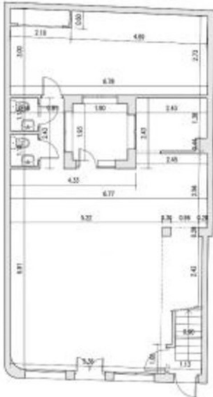
PLANTA BAJA
