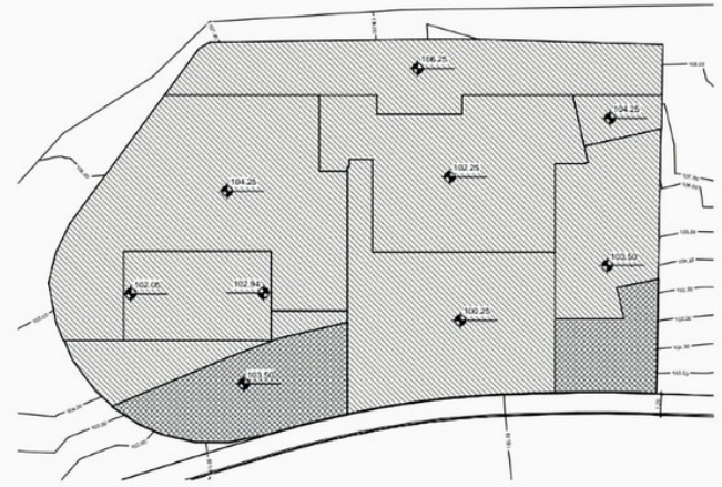
2 TOPOGRÁFICO MODIFICADO 1:150
