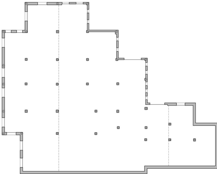
Planta cota -5.40
