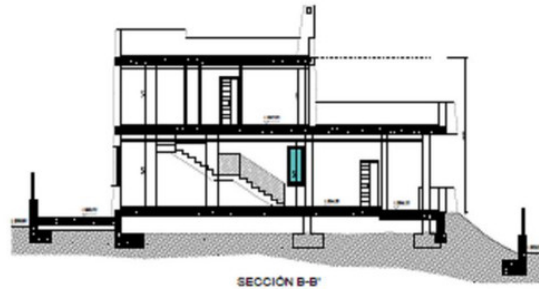
SECCIÓN B-B'
