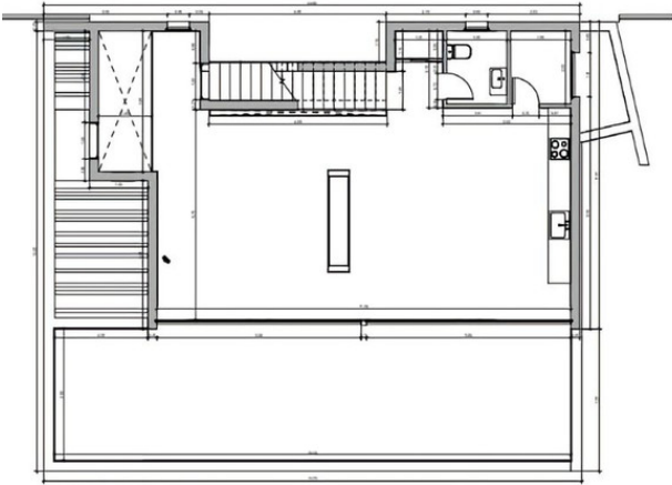
3 PLANTA ALTA - ACOTADO 1:50
