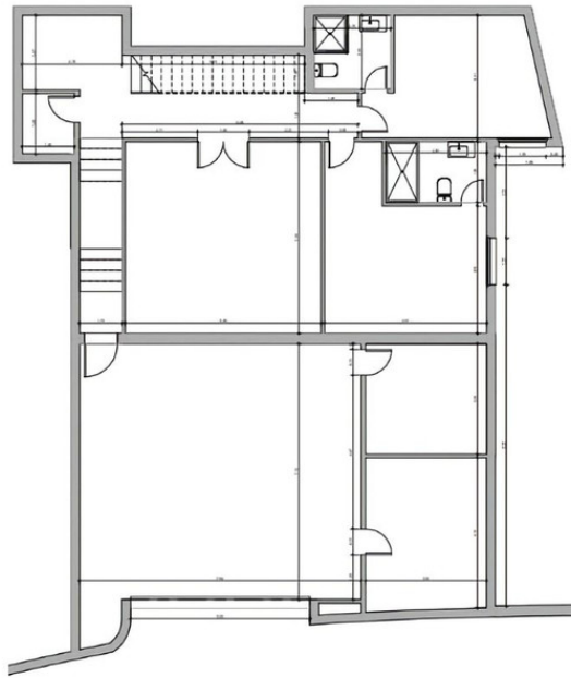
1 PLANTA SÓTANO - ACOTADO 1:50
