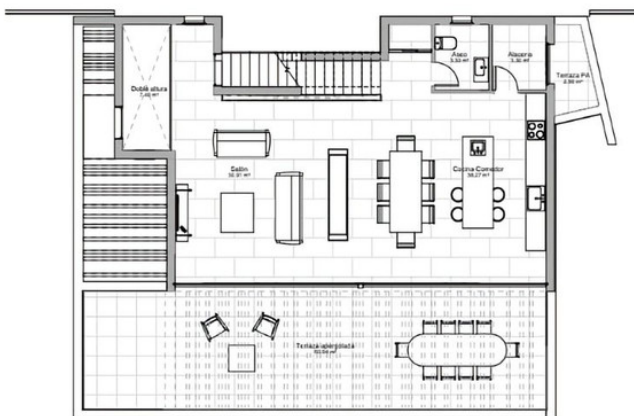
3 PLANTA ALTA 1:50
