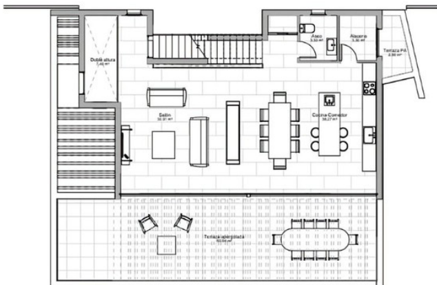
③ PLANTA ALTA 1:50
