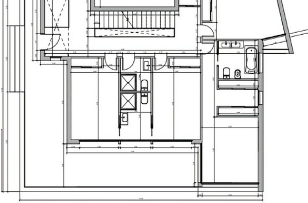
2 PLANTA BAJA - ACOTADO 1:50
