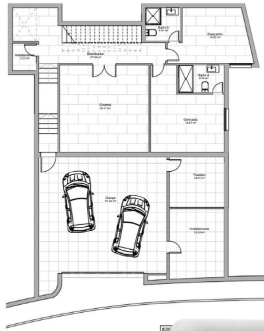
1 PLANTA SÓTANO 1:50
