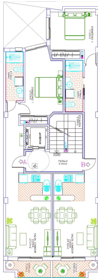
PLANTA PRIMERA
