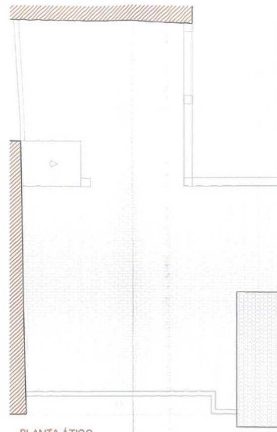
PLANTA ÁTICO
