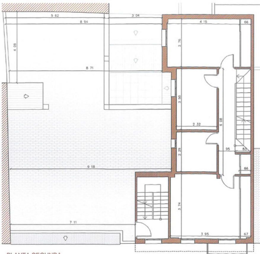
PLANTA SEGUNDA
