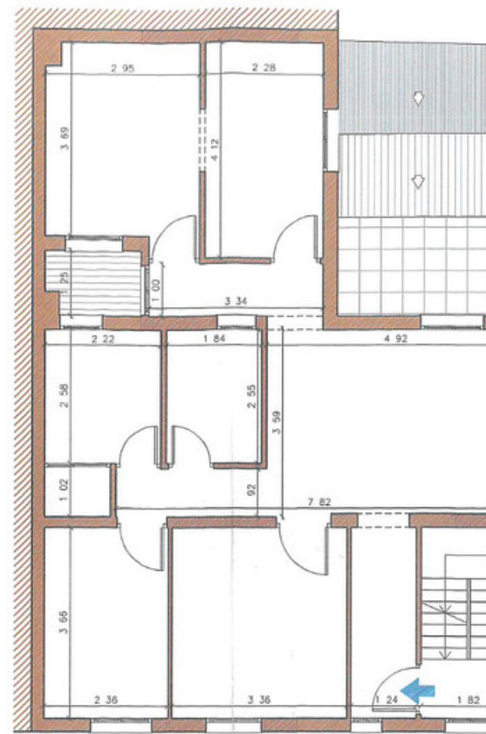
PLANTA PRIMERA
