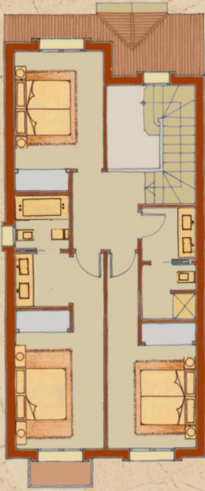
Planta Alta
