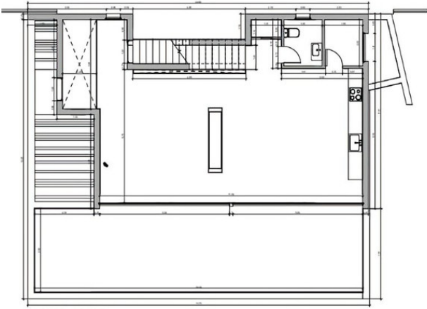
PLANTA ALTA - ACOTADO 1:50
