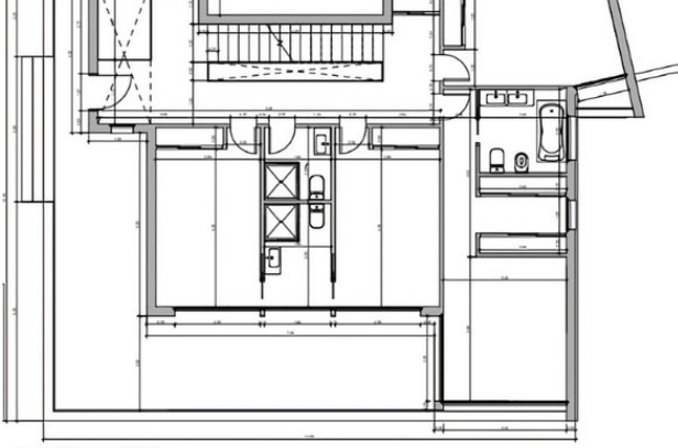
PLANTA BAJA - ACOTADO 1:50
