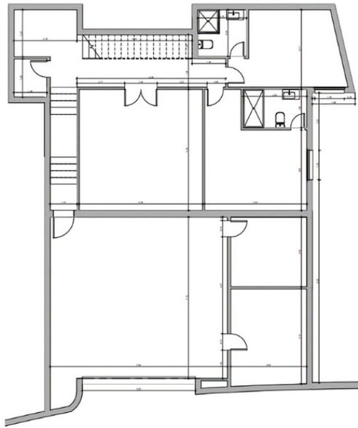
PLANTA SÓTANO - ACOTADO 1:50
