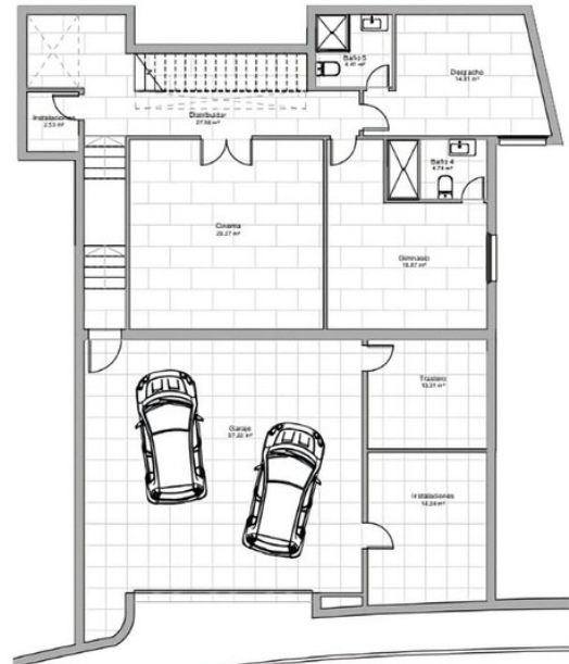
PLANTA SÓTANO 1:50
