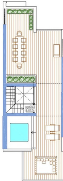
PLANTA SOLARIUM
