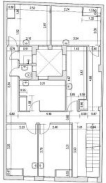
PLANTA PRIMERA
