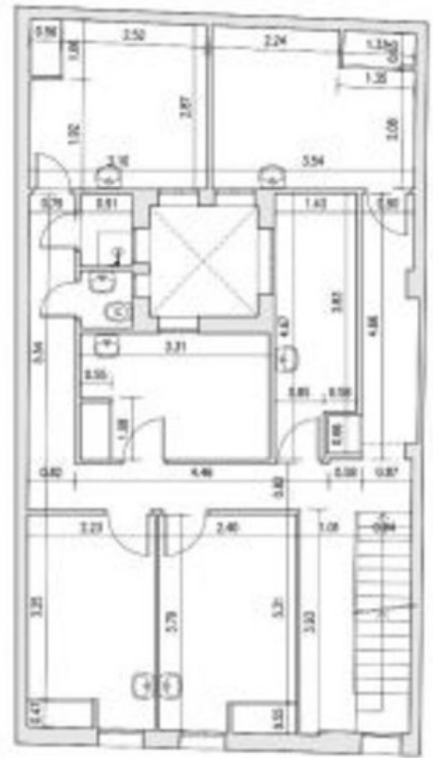
PLANTA PRIMERA
