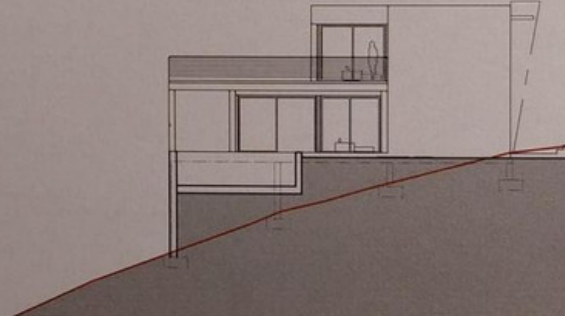
Sección B-B
