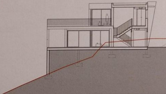
Sección A-A
