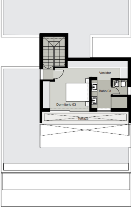
PLANTA ALTA
