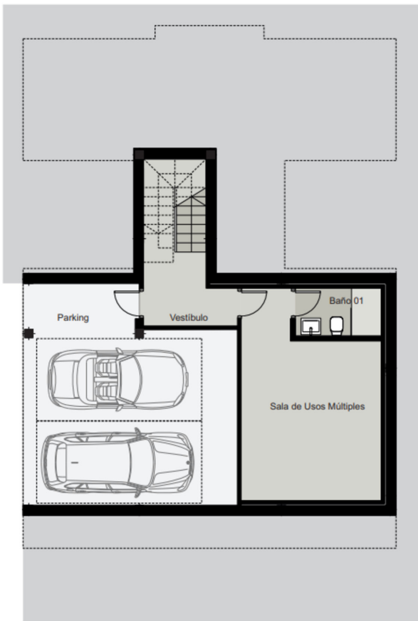
PLANTA SOTANO
