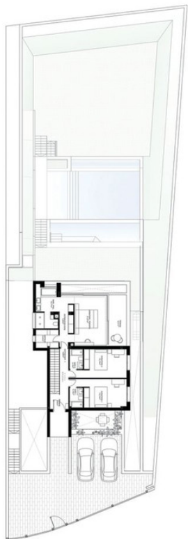
PLANTA PRIMERA FIRST FLOOR
