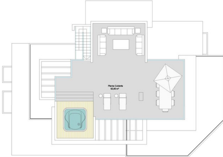
PLANTA CUBIERTAS
