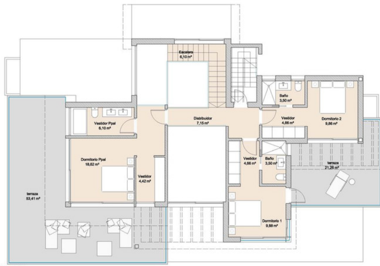
PLANTA ALTA
