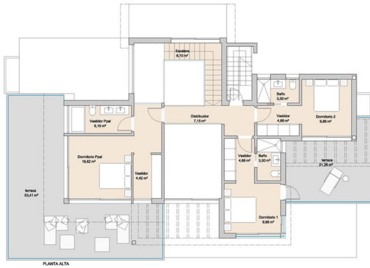
PLANTA ALTA
