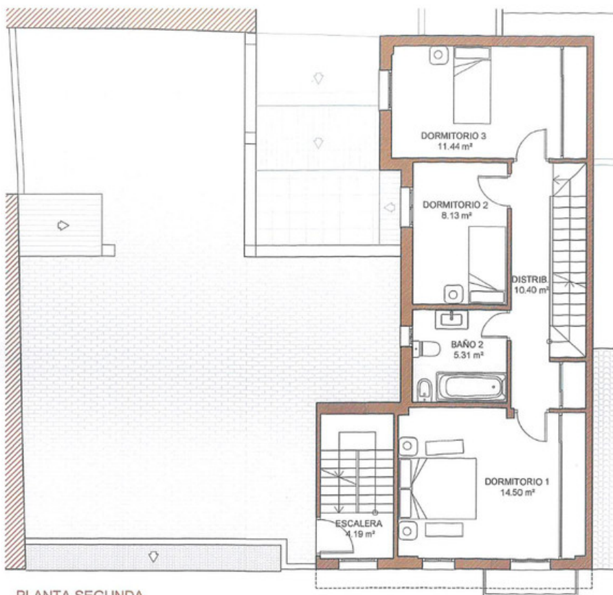
PLANTA SEGUNDA
