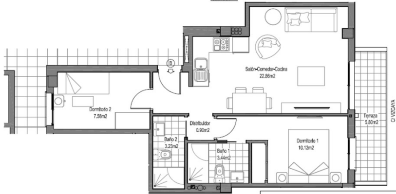
EDIFICIO DE VIVIENDAS C/ VIZCAYA, C/ RIOJA 5, FUENGIROLA, MALAGA TIPO B, PLANTA 1 2 3 4 Escala: PLANO Nº 1/50 B 1 2 3 4
