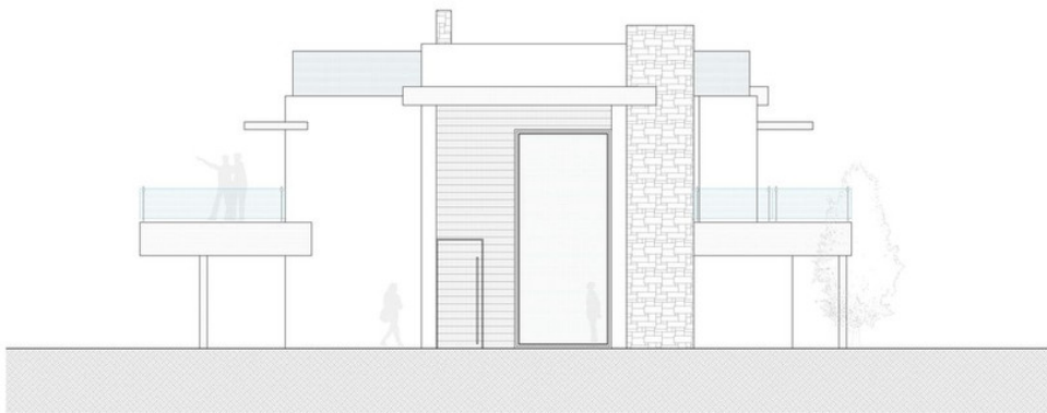
ALZADO NORTE
