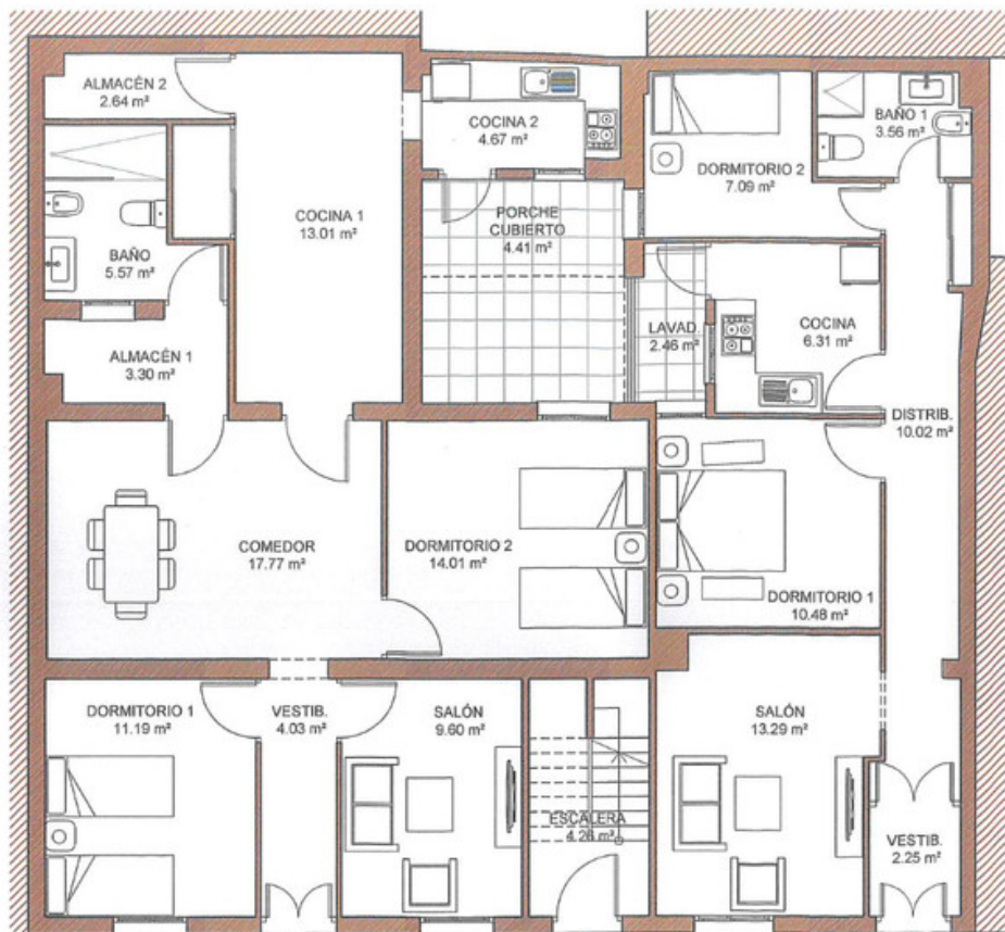
PLANTA BAJA
